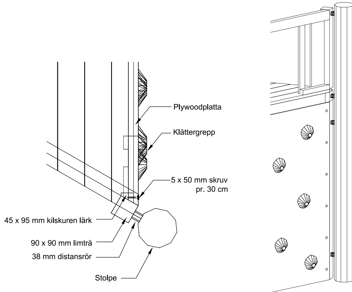
53: Monteringsprincip för klättervägg
